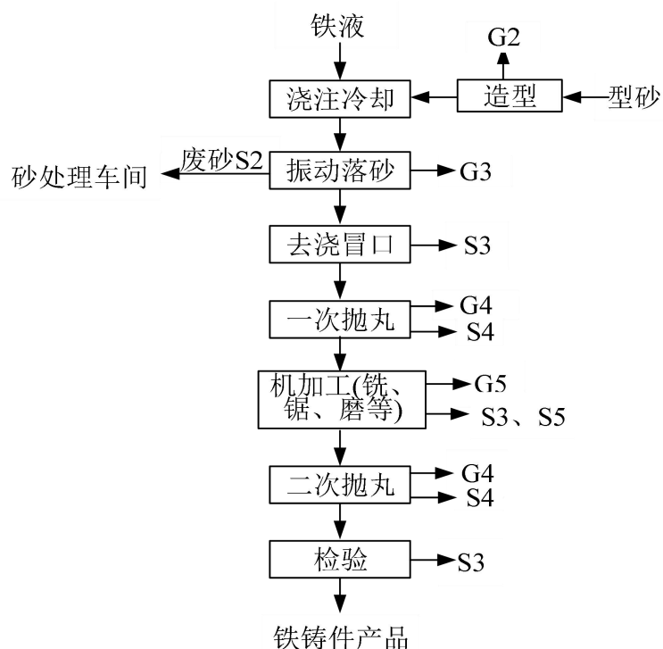
图 2-10 黑色金属浇注及后处理工序工艺流程图
