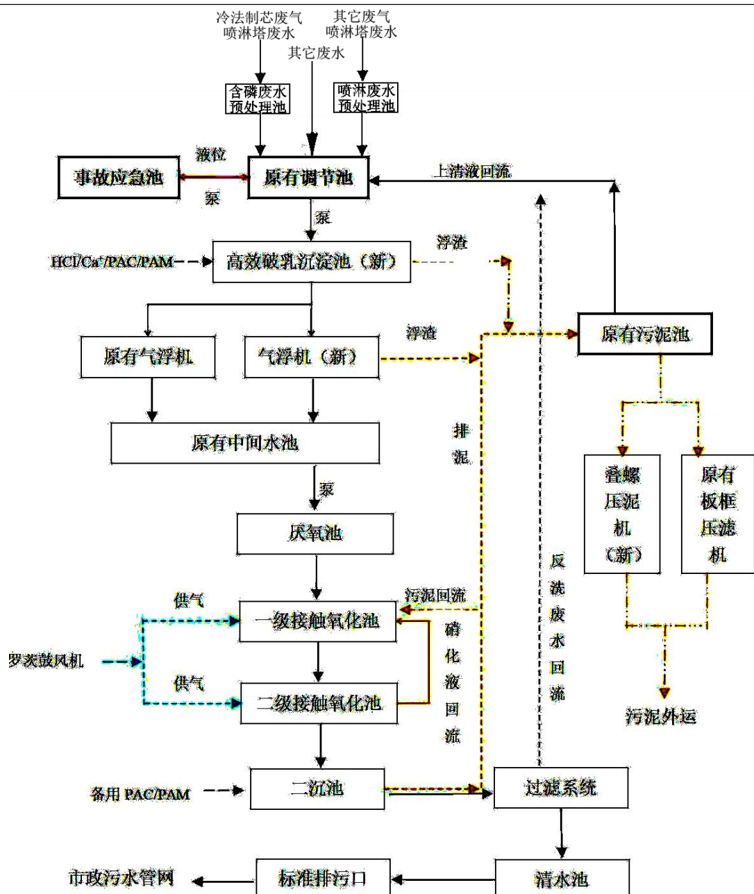
图 4-1 生产废水处理站污水处理工艺流程图
