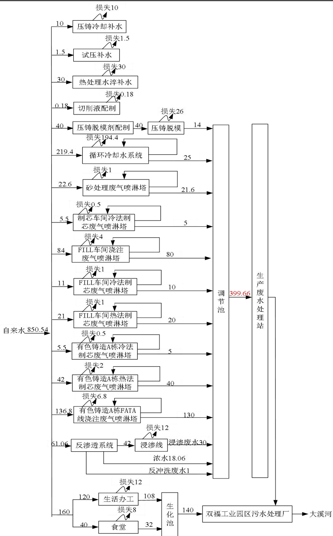
图 2-2 改扩建项目建成后全公司日最大用水量水平平衡图 m³/d
