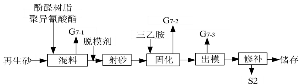
图 2-12 冷法制芯工艺流程图
