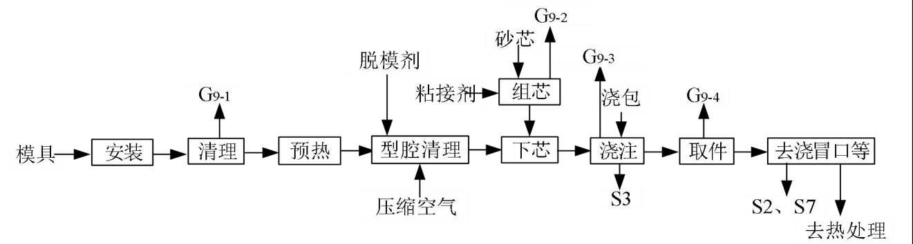
图 2-14 砂型浇注工艺流程图
