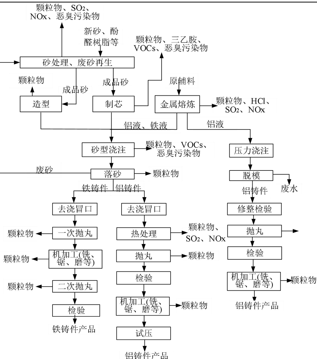
图 2-8 现有项目总生产工艺流程图
