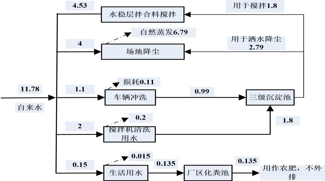
图 2-1 项目水平平衡图 单位 m³/d
