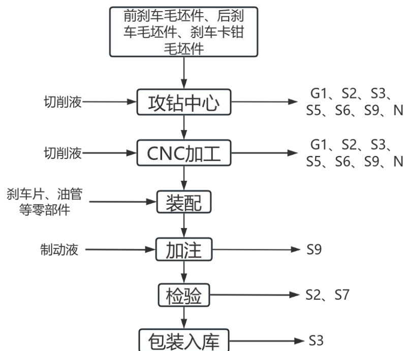
图 2.9-1 拟建项目工艺流程及产污节点图
