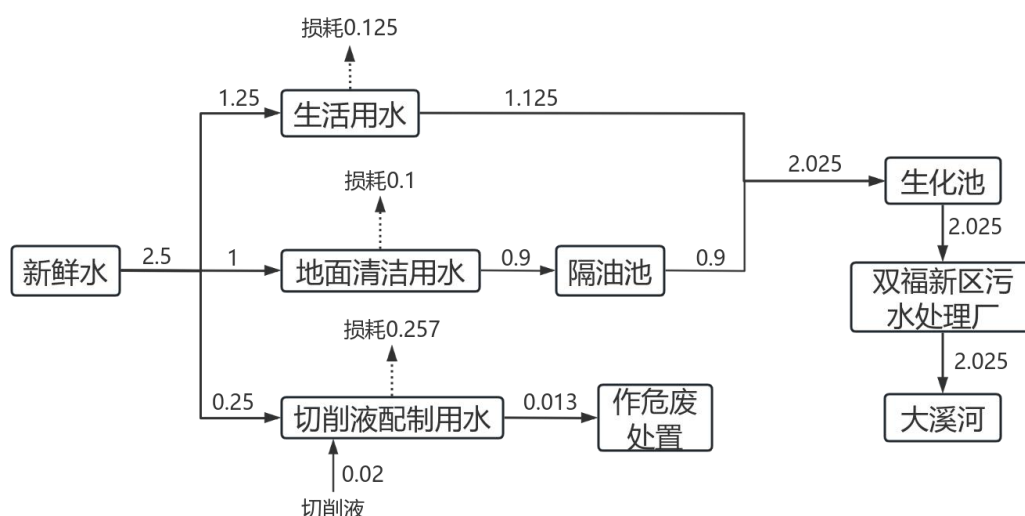
图 2.6-1 拟建项目平衡图 (m³/d)
