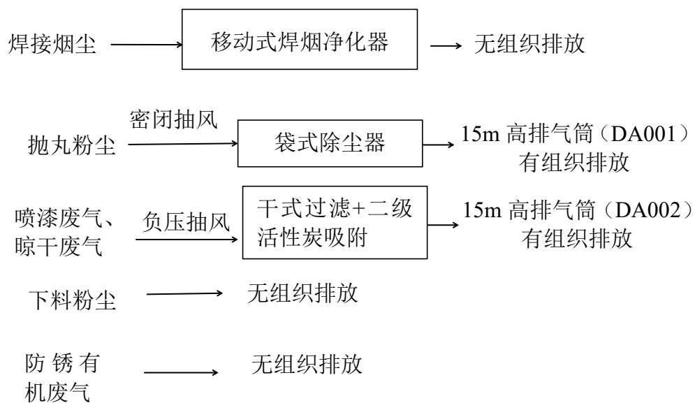
图 4.2-1 废气处理工艺流程图
