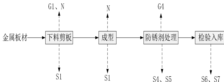
图 2.9-3 碗形塞生产工艺流程图及工艺污染环节图
