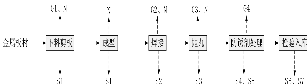
图 2.9-1 焊接支架、呼吸器、其他杂件生产工艺流程及工艺污染环节图
