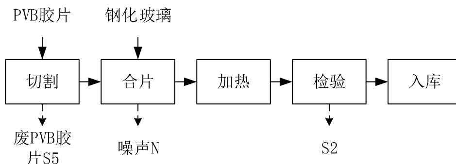
图 2.2-3 夹胶玻璃生产工艺流程及产污环节图
