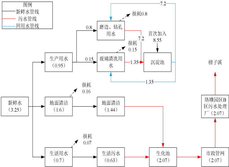
图 2.1-1 本项目水平衡图 单位：m 3 /d
