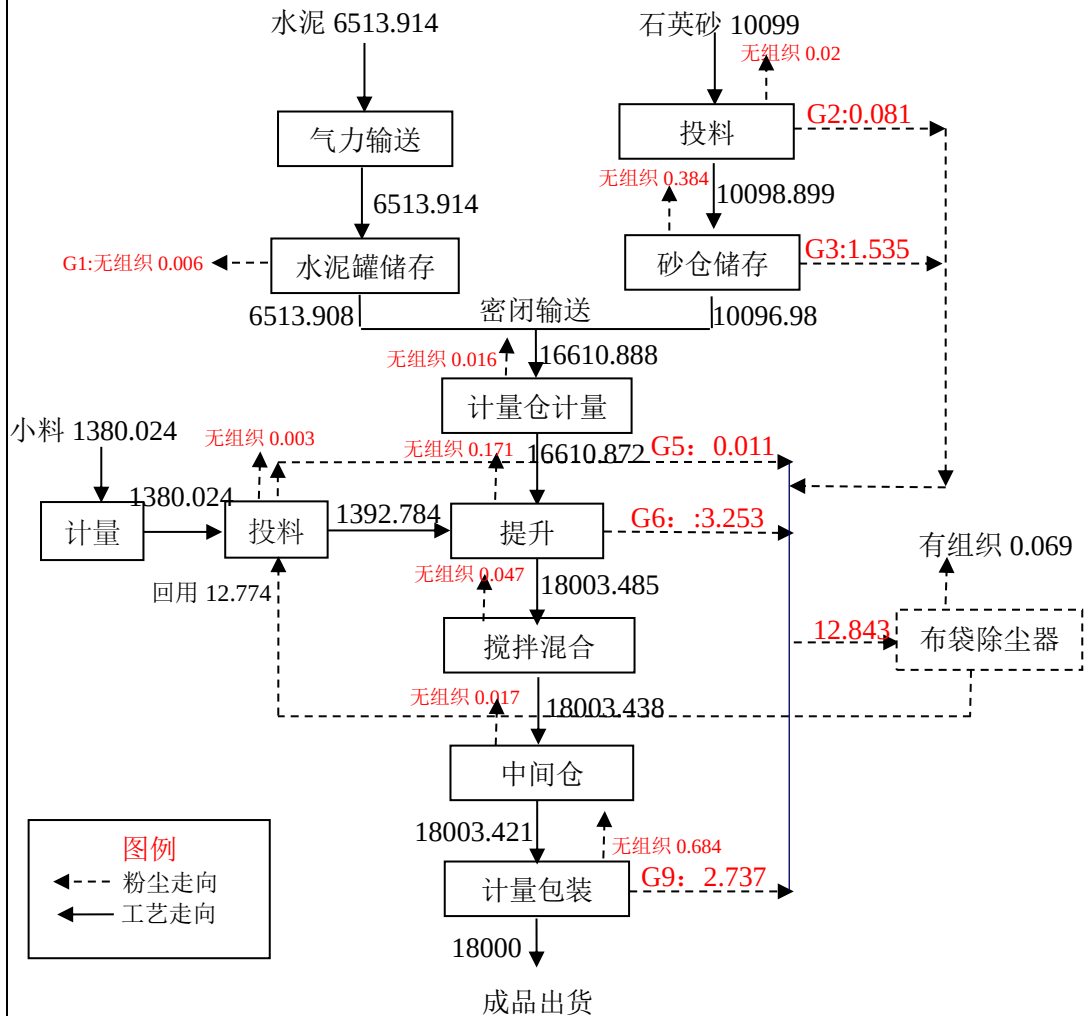
图 2.2-1 物料平衡图 单位: t/a
